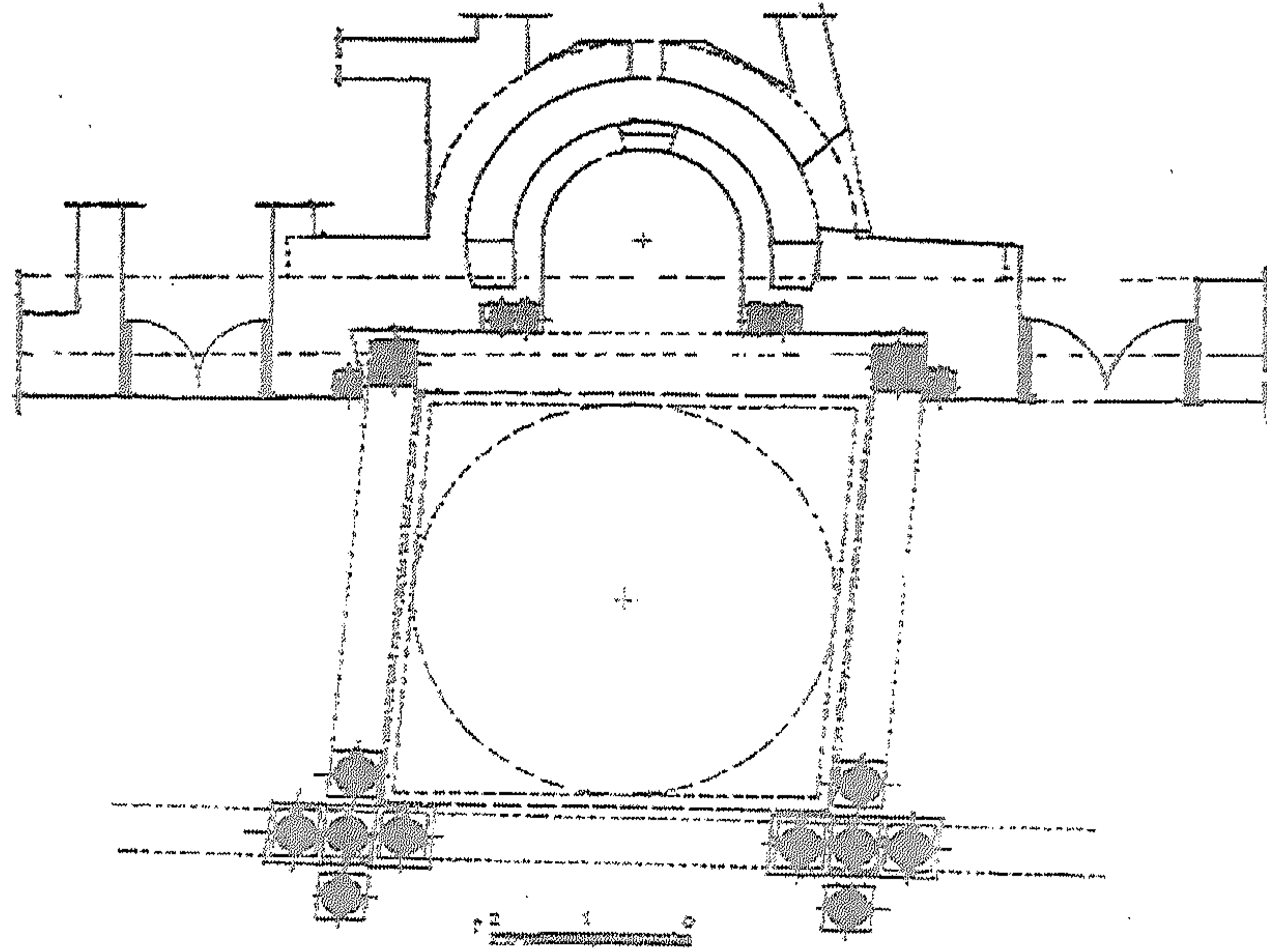
(شكل رقم ٧٨) مساقط مربع المحراب ومقطع المحرابين المتوازيين القديم والحديث بجامع الزيتونة عن د/الدولتي.
